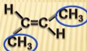
транс-изомер T_{\text{пл.}} = -105,6 \text{ }^\circ\text{C}
