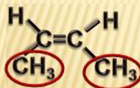
цис-изомер T_{\text{пл.}} = -138,9 \text{ }^\circ\text{C}
